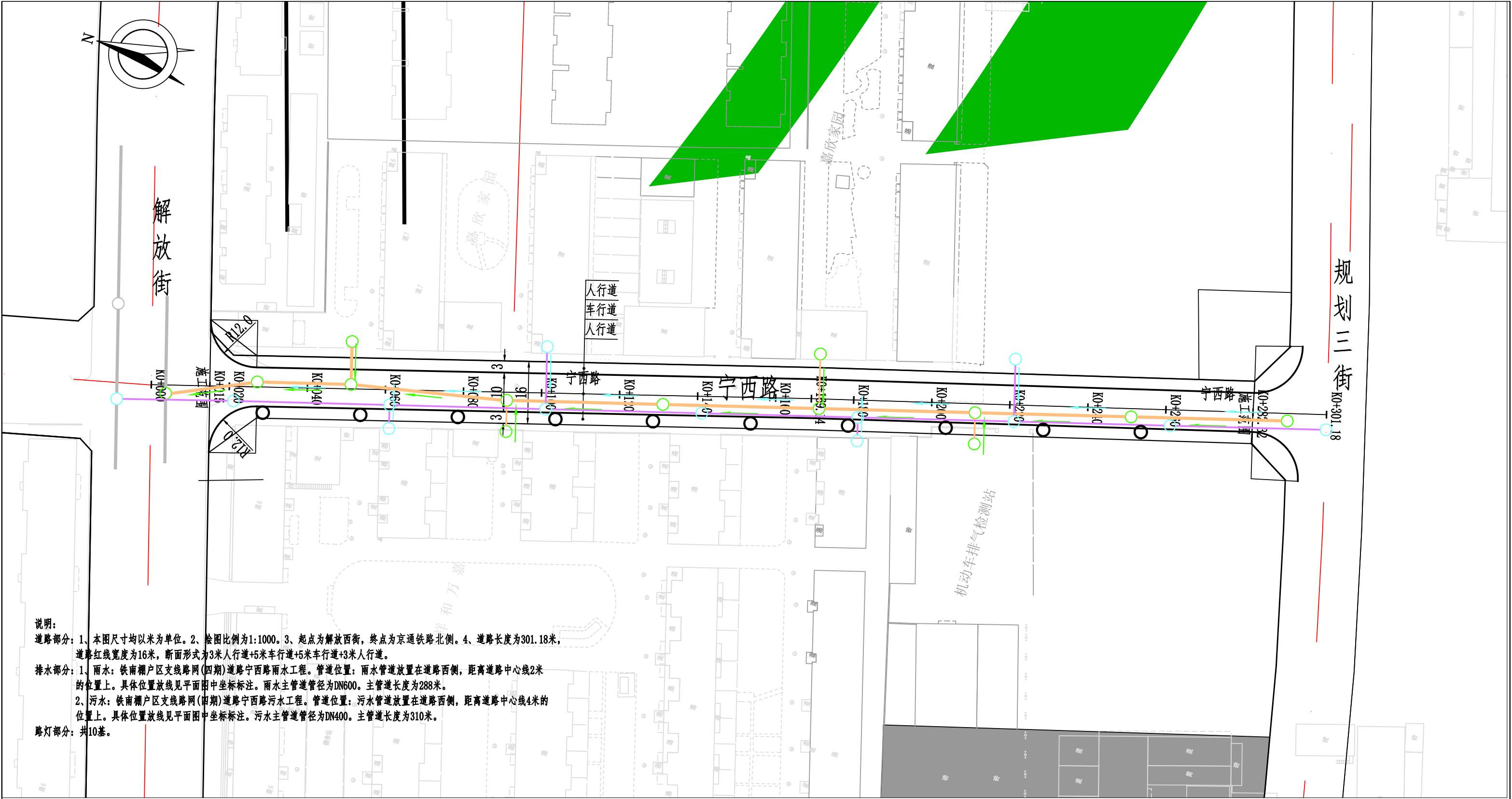
赤峰市红山城市基础设施投资有限公司赤峰市红山区铁南棚户区支线路网（四期）道路建设工程项目—宁西路（解放街—规划三街）规划总平面图（1:1000）
